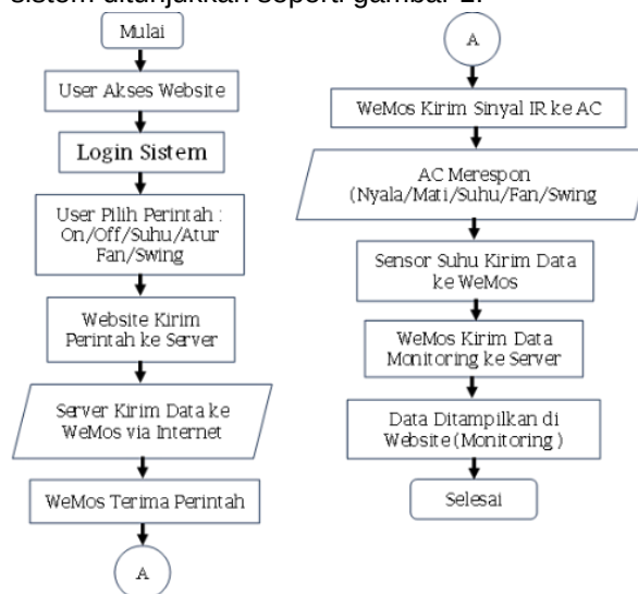
Gambar 1. Daigram Alir Sistem
