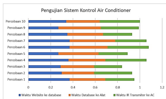
Gambar 13. Grafik pengujian sistem kontrol air conditioner
