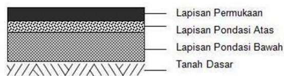
Gambar 2. Lapisan Jalan
