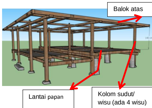
Gambar 4. Pemasangan Balok dan Kolom
