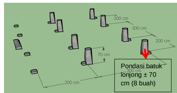
Gambar 3. Pemasangan Pondasi
