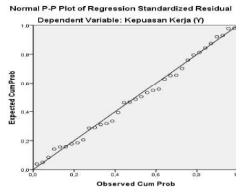
Gambar 1 Uji Normalitas
